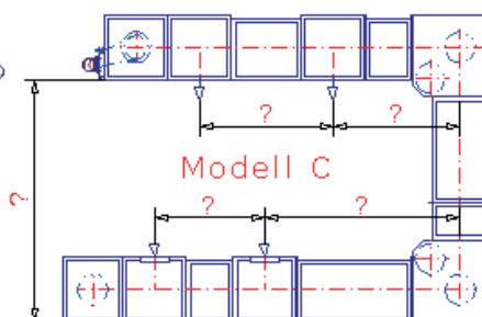
Aufstellungsbeispiele
